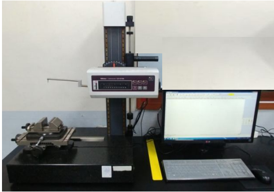
형상 측정기
