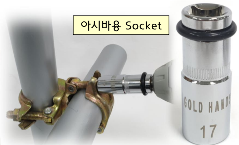
롱 비트 소켓 실 현장 사용 모습
